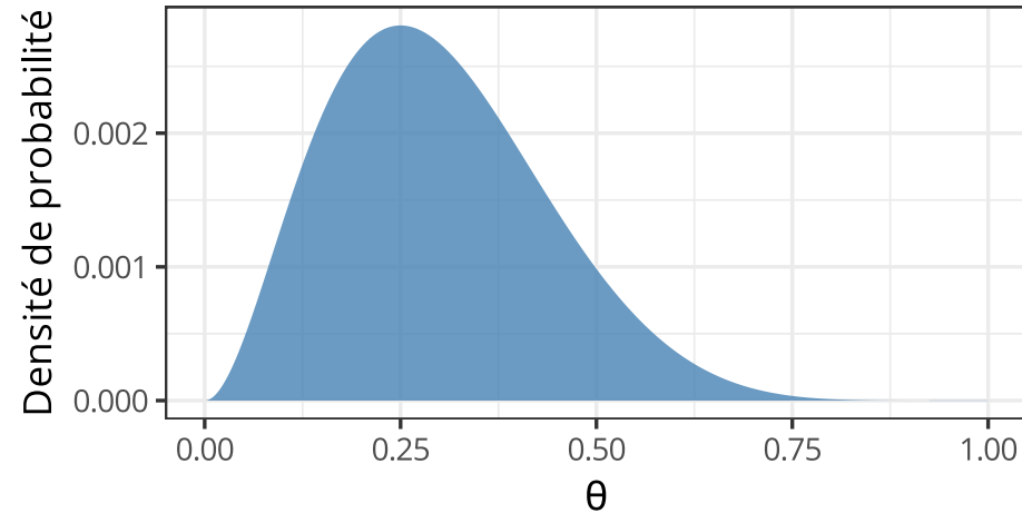
Posterior distribution
