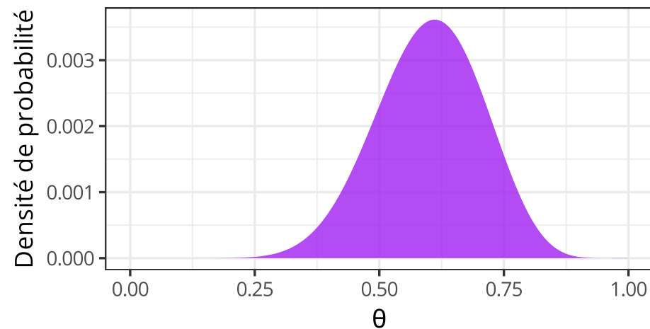
Posterior distribution
